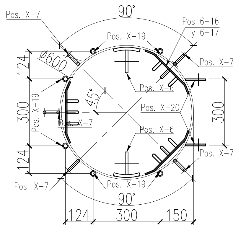
CORTE G-G
