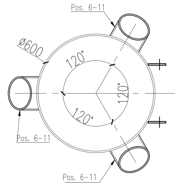
CORTE E-E
