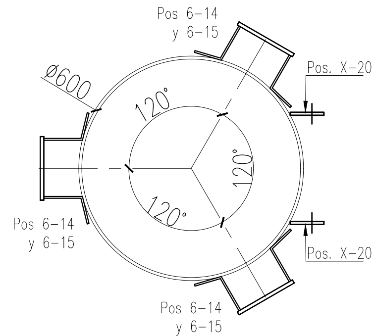
CORTE F-F
