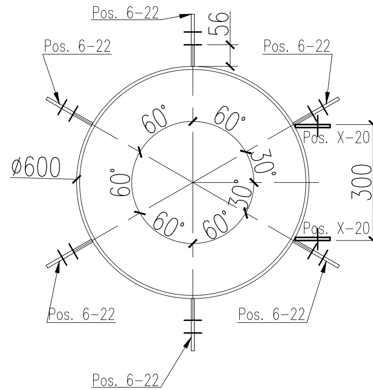
CORTE D-D
