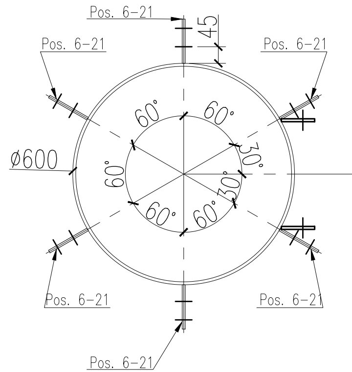
CORTE C-C
